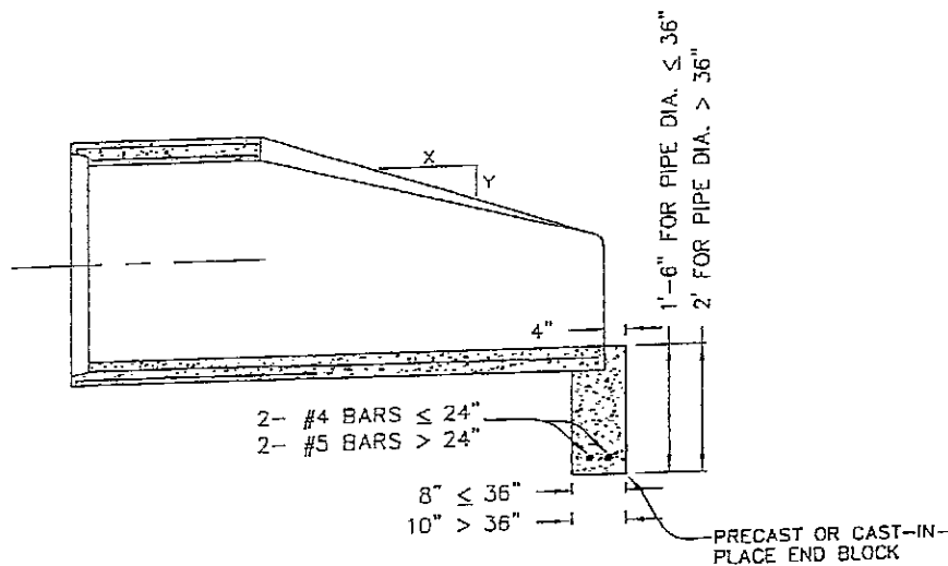
LONGITUDINAL SECTION
